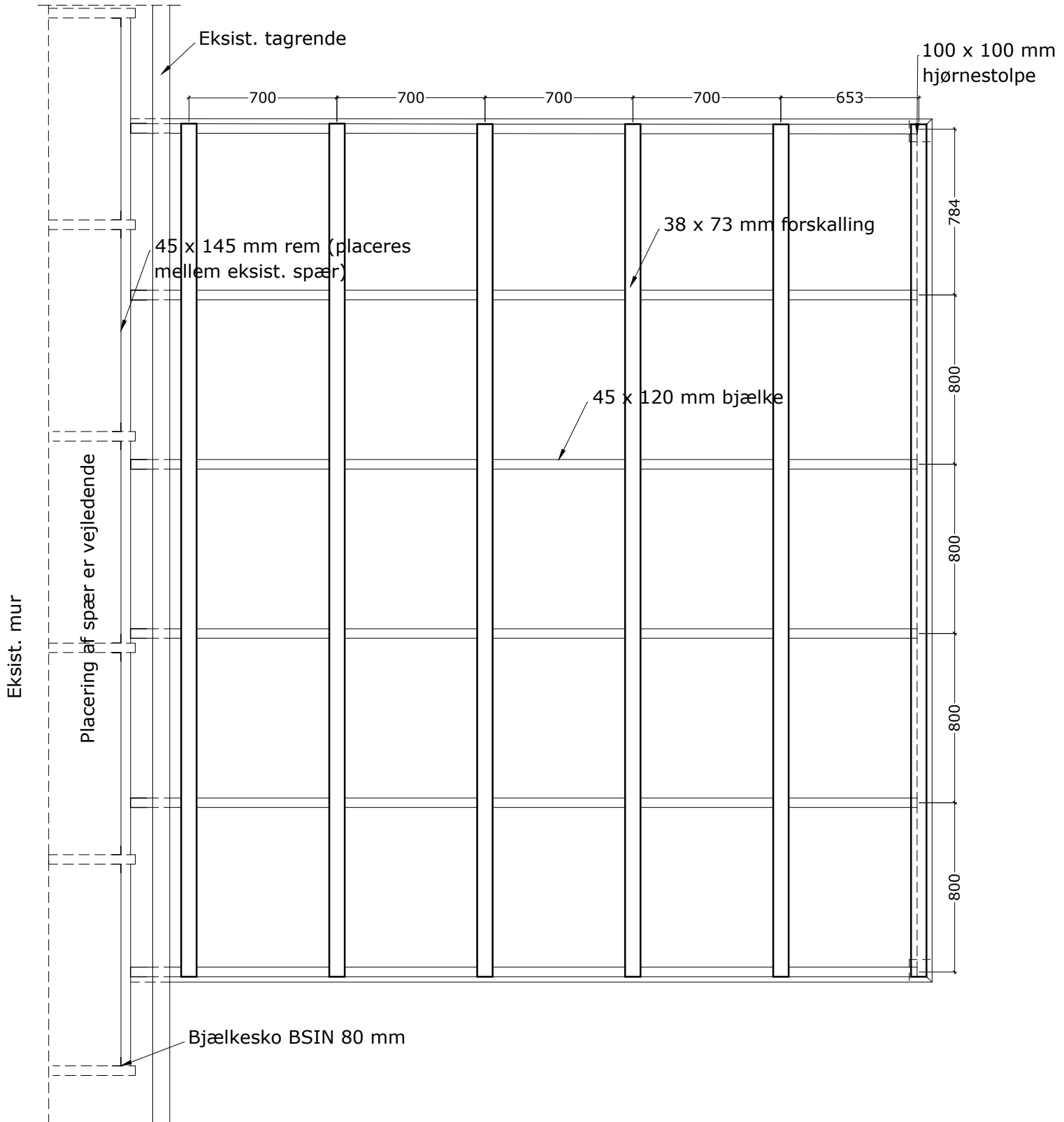
OV1 ALM. - SPÆRPLAN 1:25
