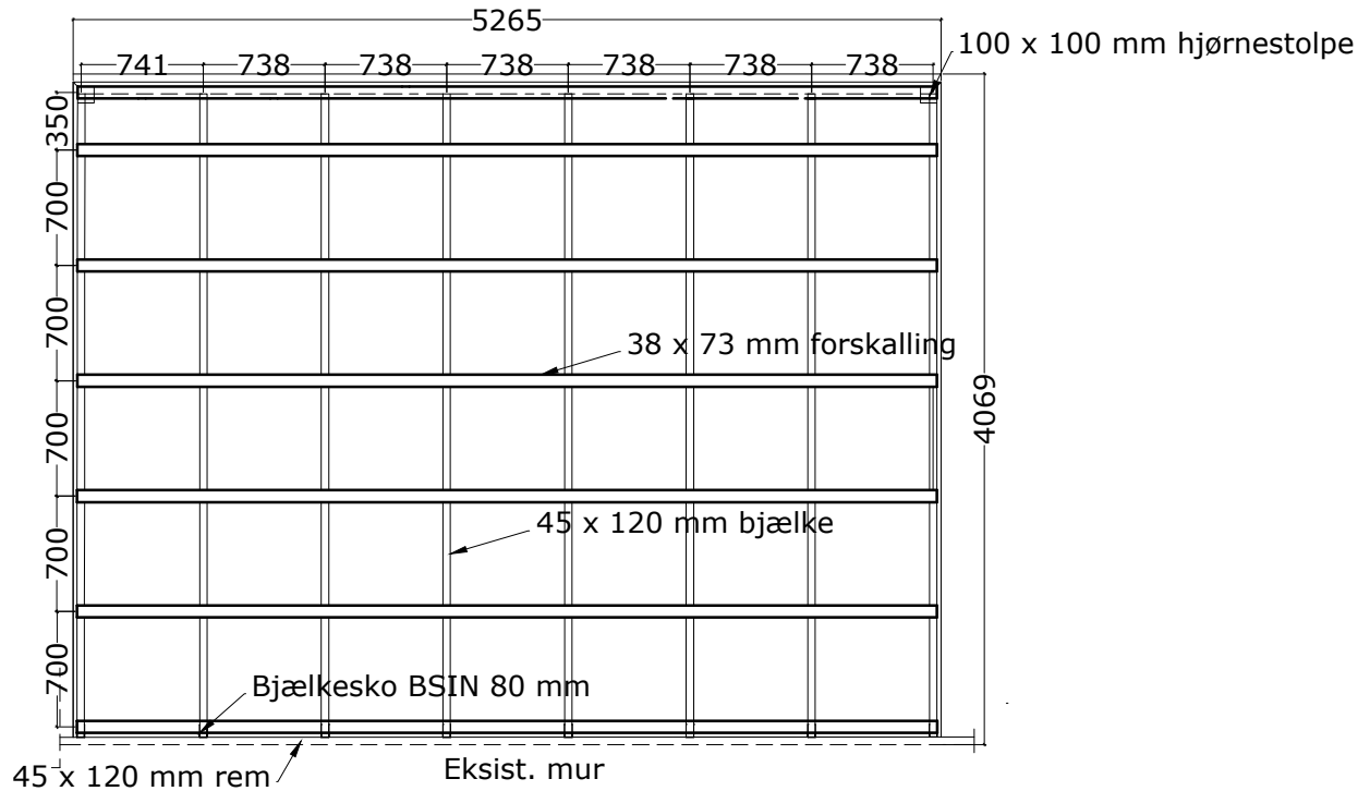
OV2 STOR. - SPÆRPLAN 1:50
