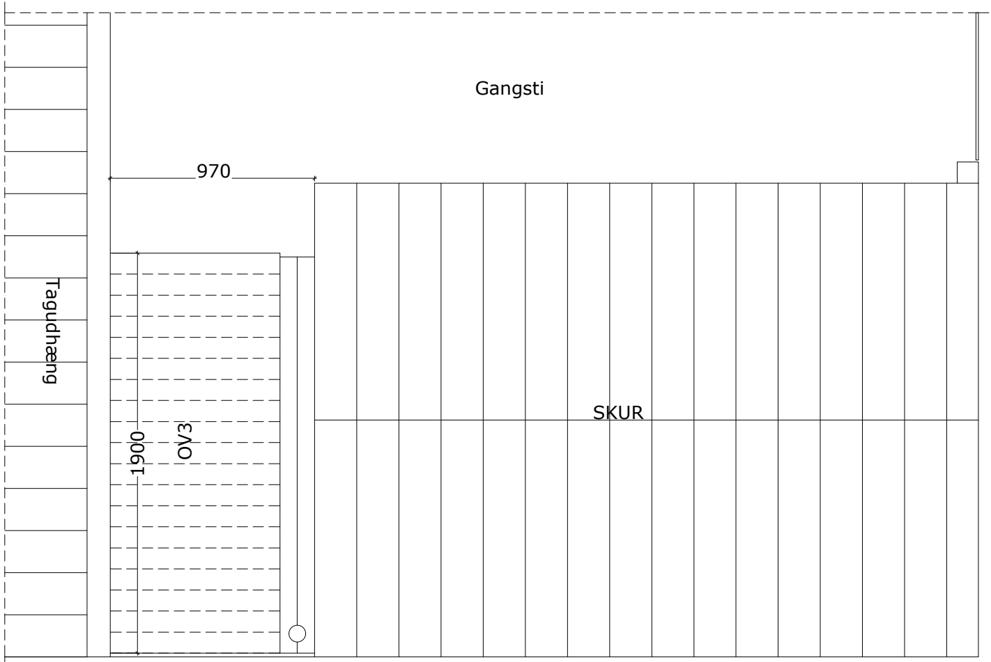
PLAN 1:25
